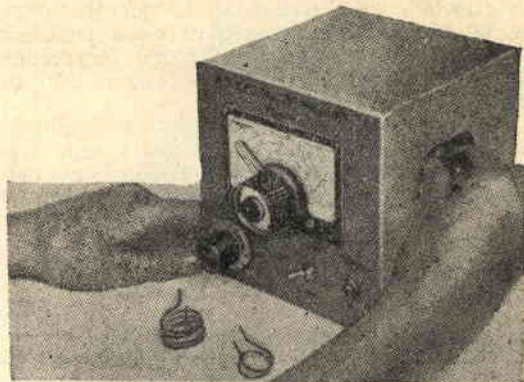
Fig. 6. — Prototipo del radio-esploratore.
