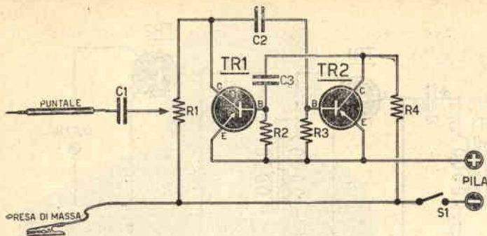
Fig. 3. - Schema elettrico del Multivibratore.
