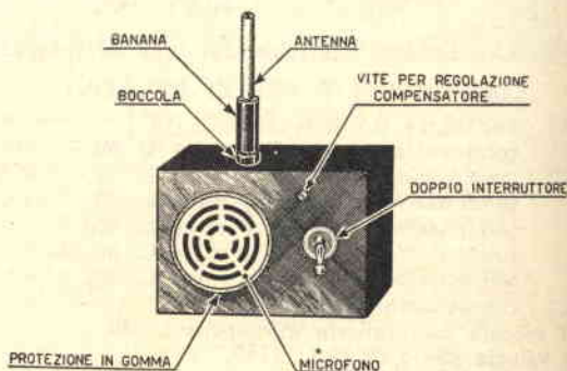
Fig. 3. - Come appare il monovalvolare alloggiato all'interno di una custodia di ridottissime dimensioni.
