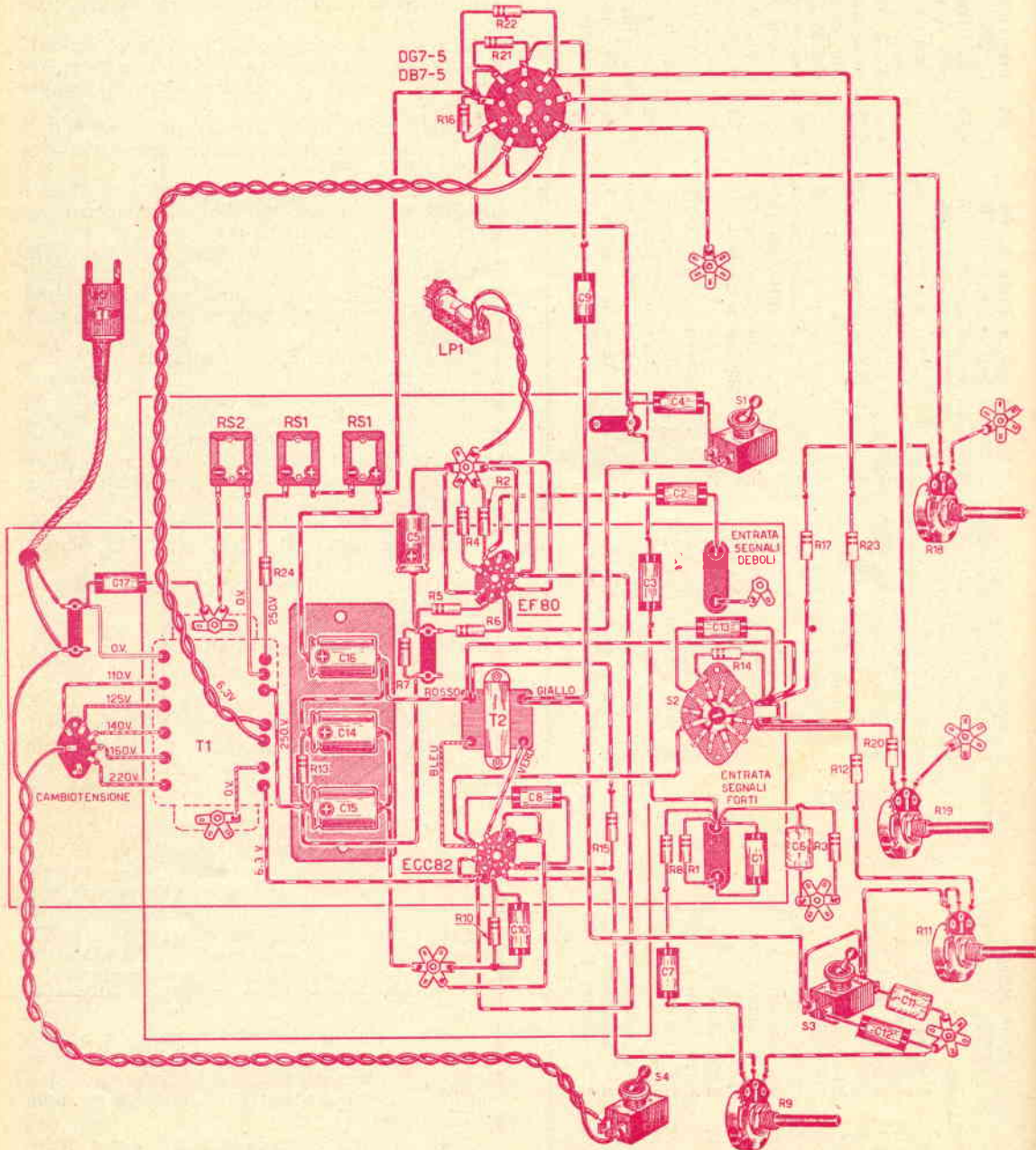
Fig. 2. - SCHEMA PRATICO DELL'OSCILLOGRAFO.
