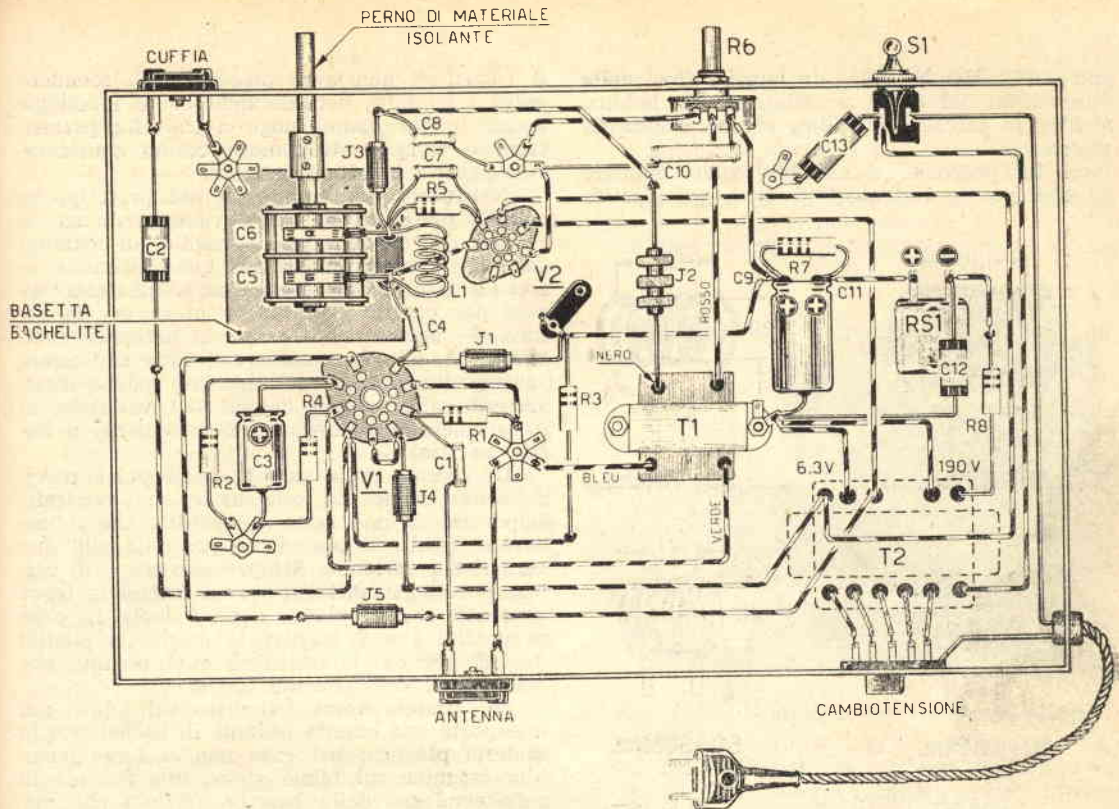
Fig. 2. — Schema pratico del radio-esplore.
