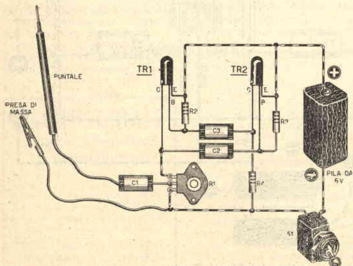
Fig. 4. - Schema pratico del Multivibratore.
