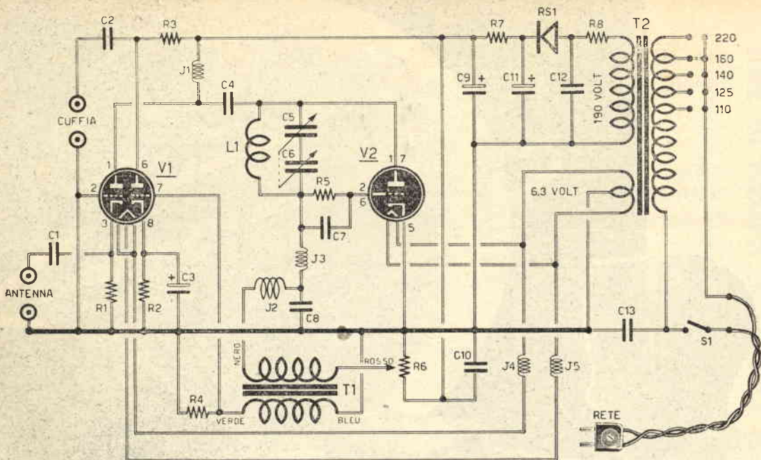
Fig. 1. — Schema elettrico del radio-esploratore.
