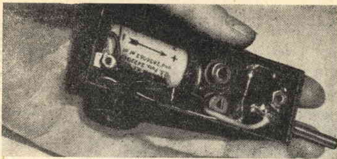
Fig. 5. - Appaiono evidenti le ridotte dimensioni di ingombro del Multivibratore a due transistori.
