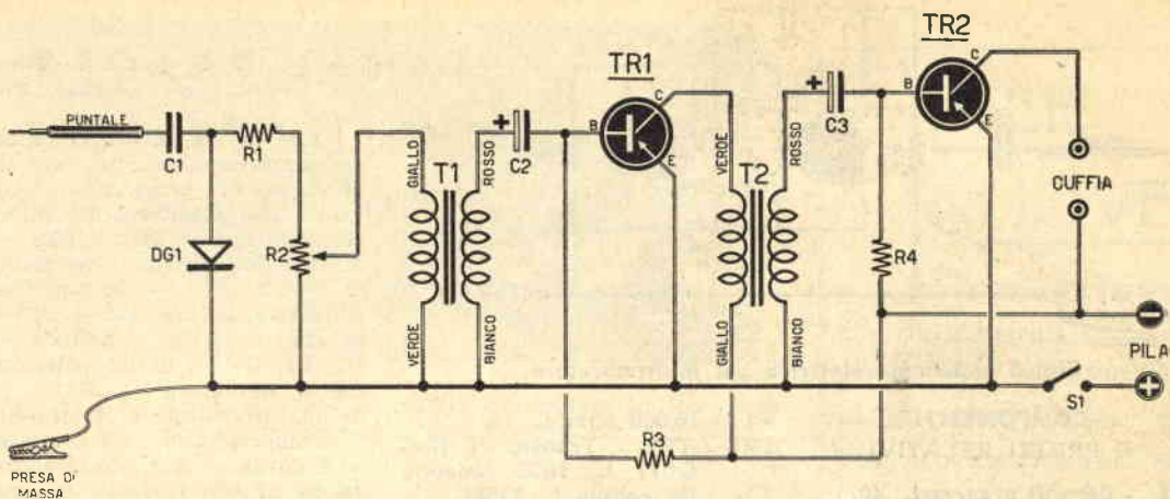
Fig. 1. - Schema elettrico del Signal Tracer.
