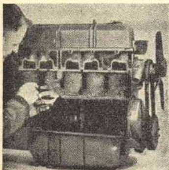
Fig. 2. — Le incrostazioni che si accumulano sulle pareti del monoblocco a contatto con l'acqua di raffreddamento sono talvolta di considerevole spessore.
