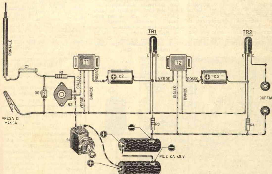
Fig. 2. - Schema pratico del Signal Tracer.
