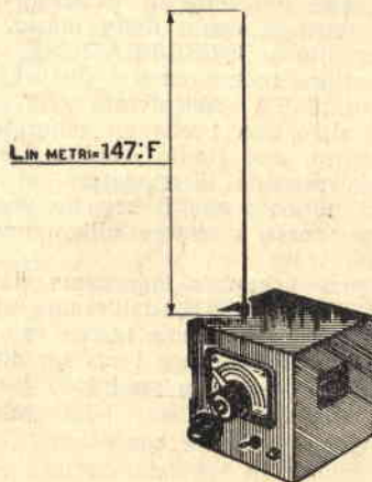
Fig. 4. — Antenna a stilo.
