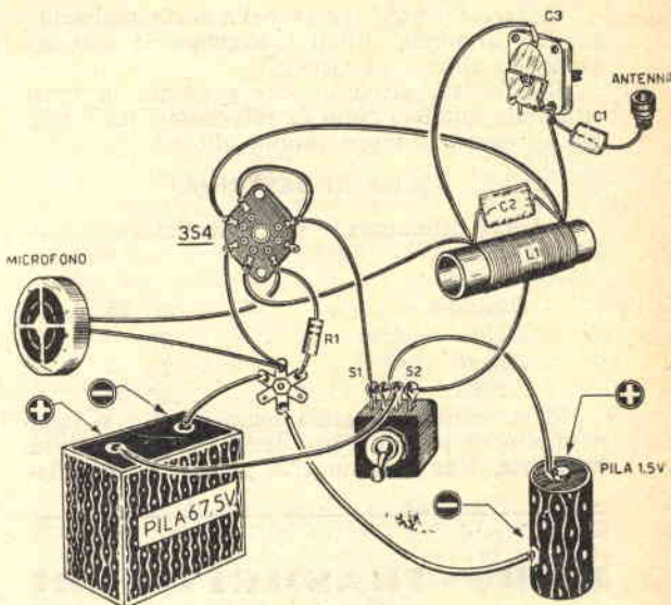
Fig. 5. - Schema pratico del monovalvole.
