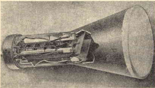
Fig. 3. — Tubo RC tipo DG7/5
