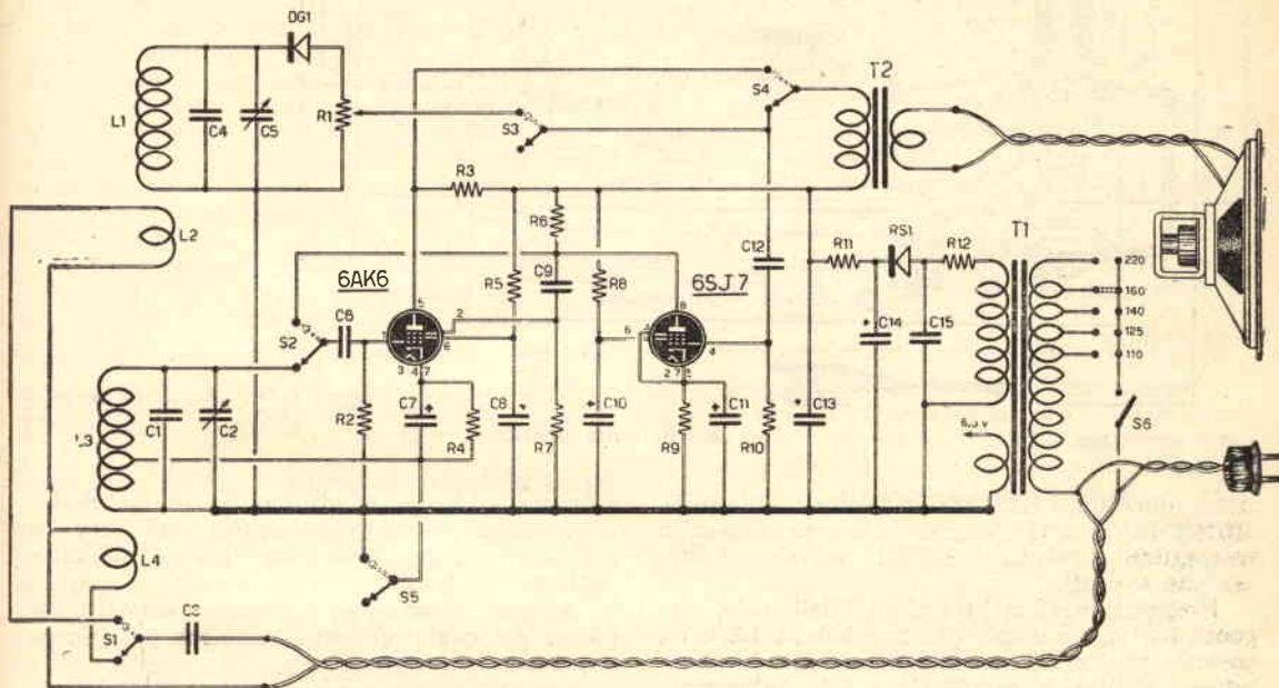
Fig. 1 - Schema elettrico
