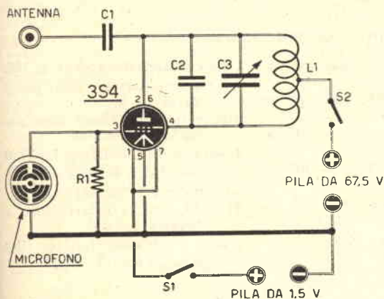
Fig. 1. - Schema elettrico del monovalvolare.
