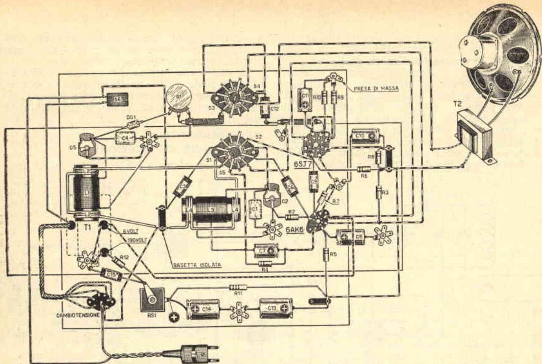
Fig. 2 - Schema pratico
