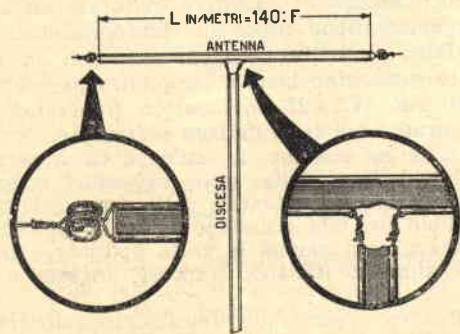
Fig. 5. — Antenna a dipolo.
