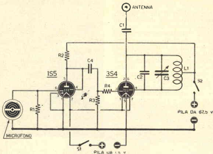
Fig. 2. - Schema elettrico del bivalvolare
