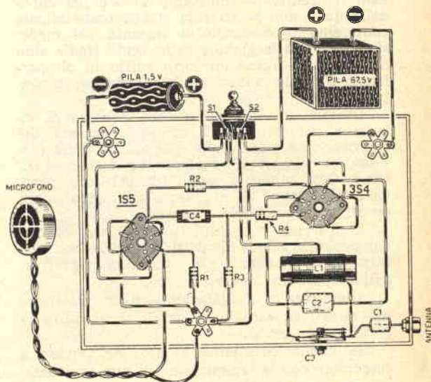
Fig. 6. - Schema pratico del bivalvole.
